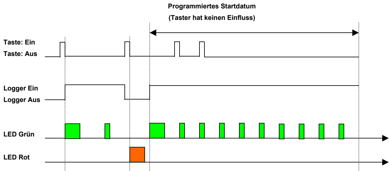
Timing Diagram: Datenlogger THC/TIC im Start/Stop-Modus
